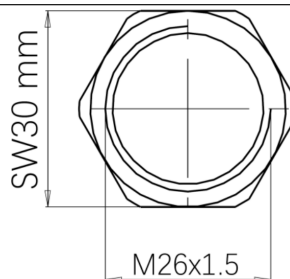
配件螺母
