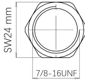
配件螺母
