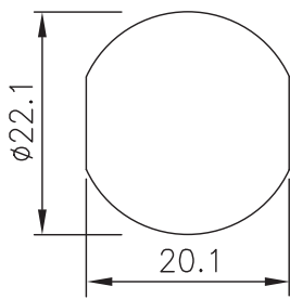
开孔尺寸
