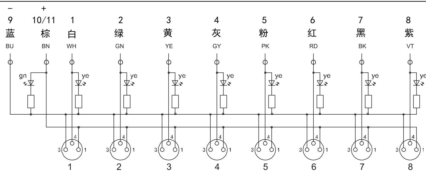
PNP接线图
