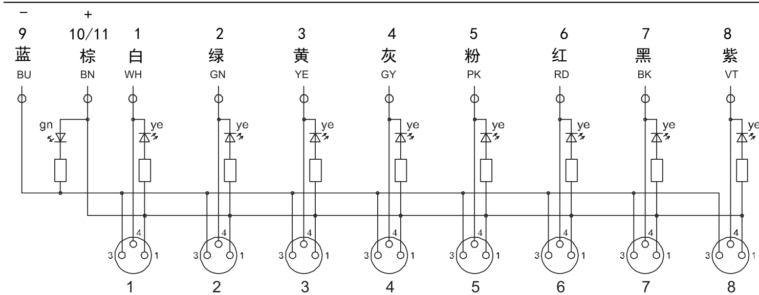
NPN接线图
