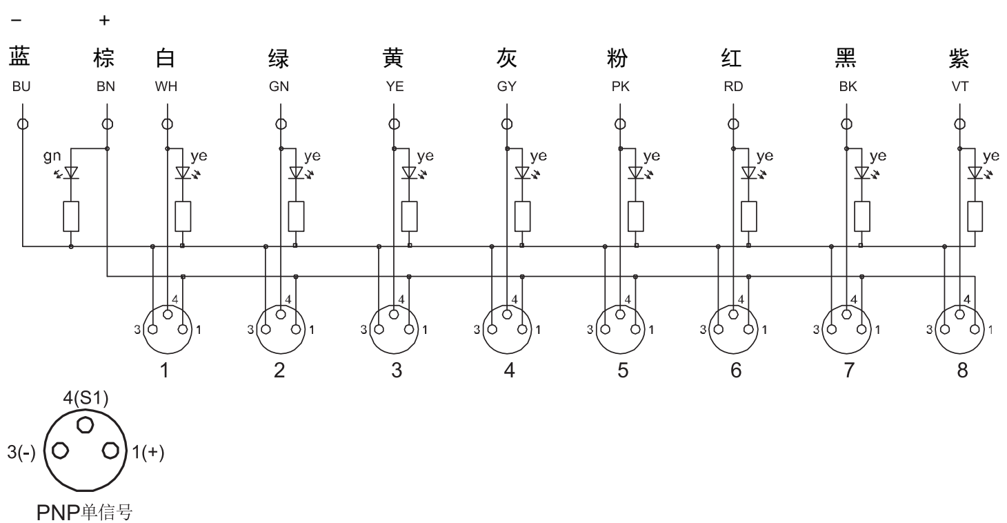
PNP接线图
