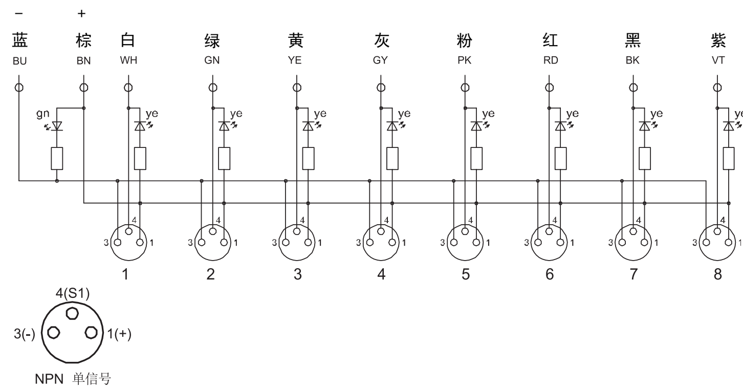
NPN接线图
